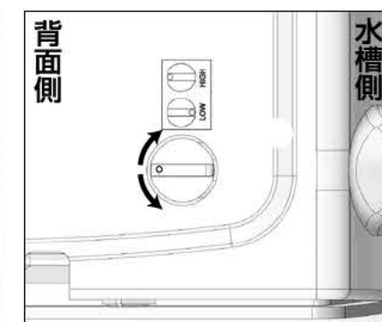
バルブを回転させて流量を調節
